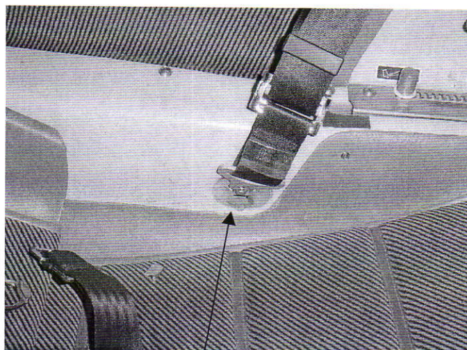
Ferrure fixation harnais
